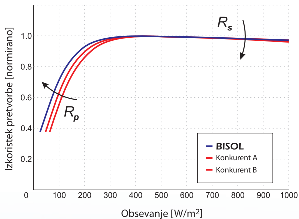
Relativni izkoristek pretvorbe
