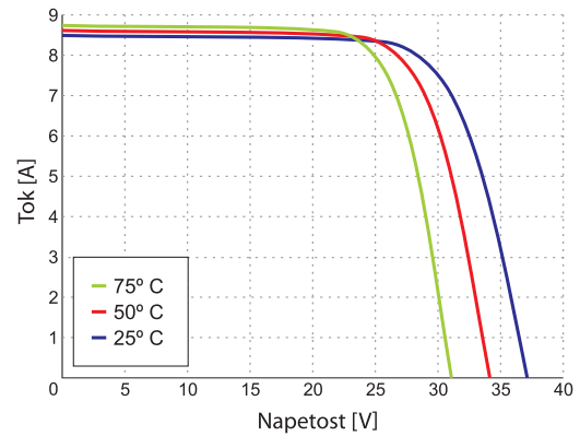
I-U krivulja pri različnih temperaturah celic
