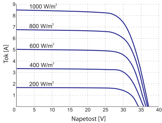
I-U krivulja pri različnih osvetlitvah
